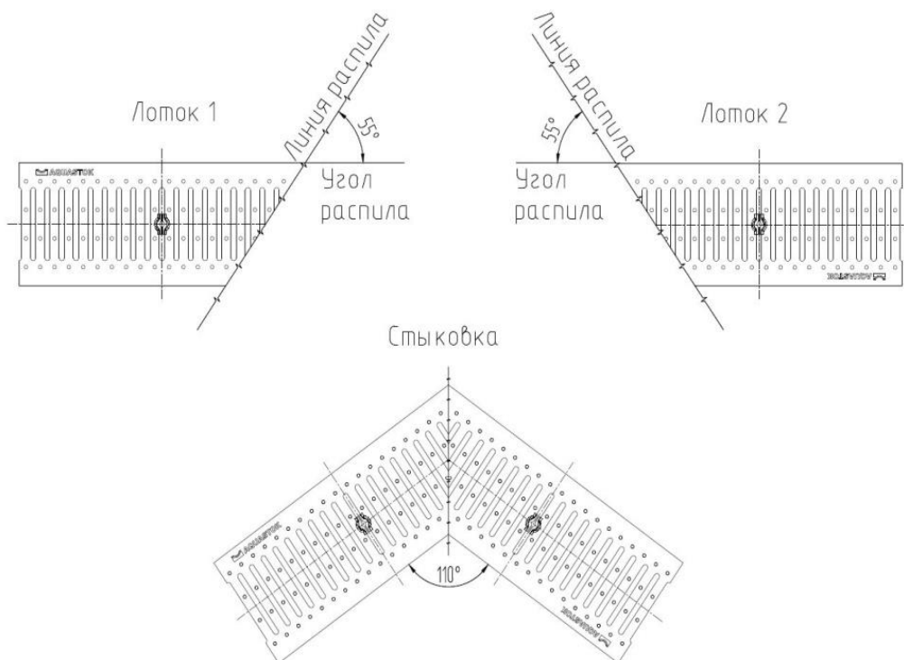
Рис. 10 – Пример стыковки распиленных лотков.
